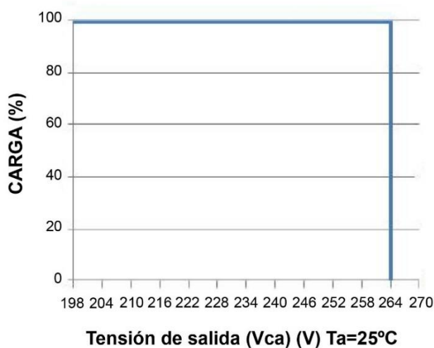
Carga vs Tensión de Salida
