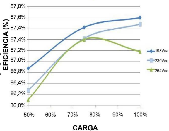
Eficiencia vs Curva de Carga
