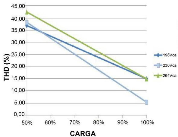
Curva Distorsión Armónica
